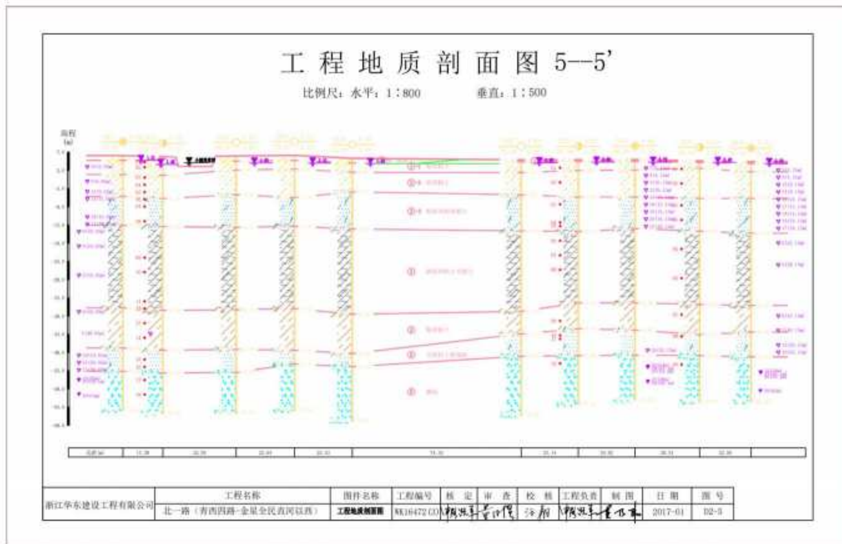
图 3-3 工程地质剖面
