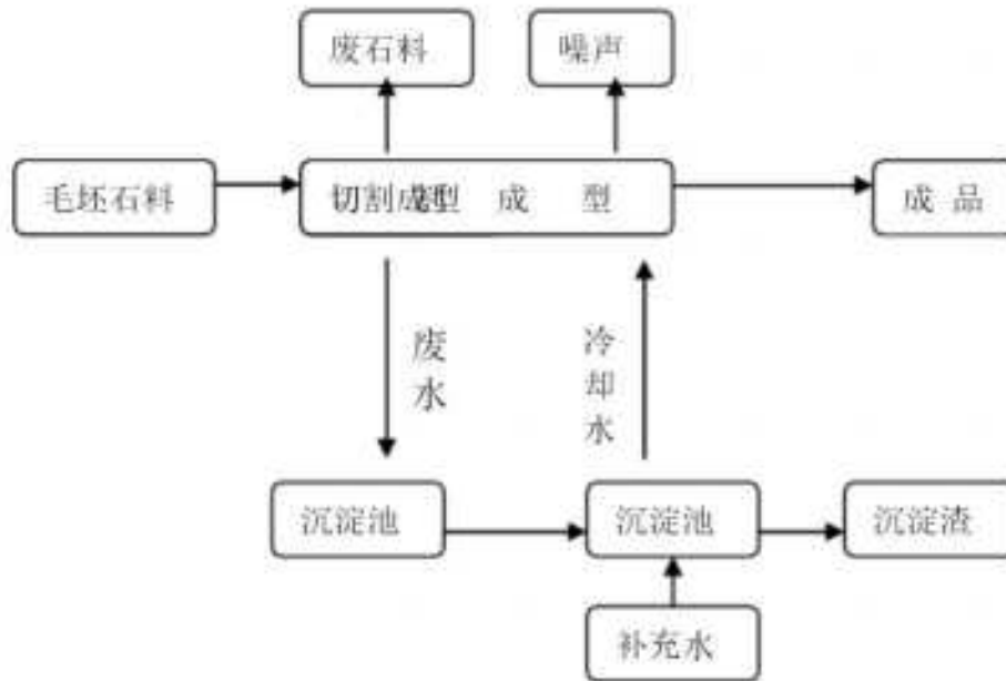
图 3-9 类比石材加工生产流程及产废
